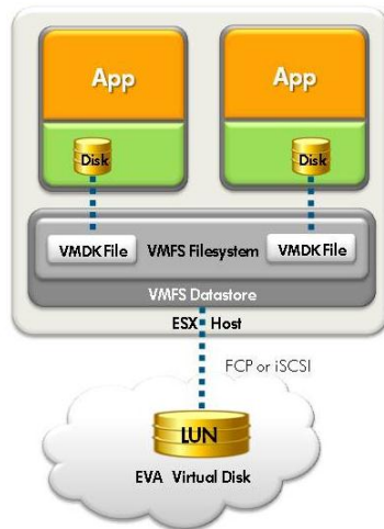
Figure 11. VMFS datastore
